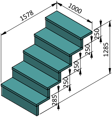
Schody X-AIR 5-stupňové pro hloubku 1,5 m pravé provedení: 2B04-01-SD085 levé provedení: 2B04-01-SD075
