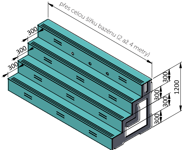
Schody obdélníkové 4-stupňové pro hloubku 1,5 m přes celou šířku bazénu (2 až 4 metry)
