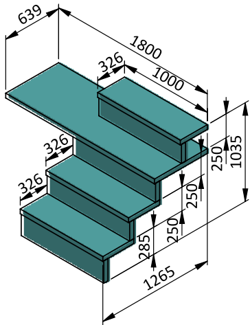
Schody X-AIR PLUS 4-stupňové pro hloubku 1,2 m pravé provedení: 2B04-01-SD076 levé provedení: 2B04-01-SD086
