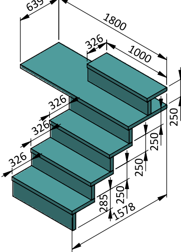
Schody X-AIR PLUS 5-stupňové pro hloubku 1,5 m pravé provedení: 2B04-01-SD077 levé provedení: 2B04-01-SD087
