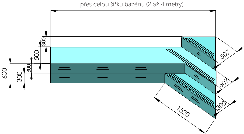
Schody rovné přes roh s lavicí 3-stupňové pro hloubku 1,2 m přes celou šířku bazénu (2 až 4 metry)
