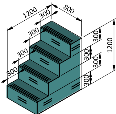
Schody obdélníkové v rohu 4-stupňové pro hloubku 1,5 m pravé provedení: 2B04-01-SD129 levé provedení: 2B04-01-SD130
