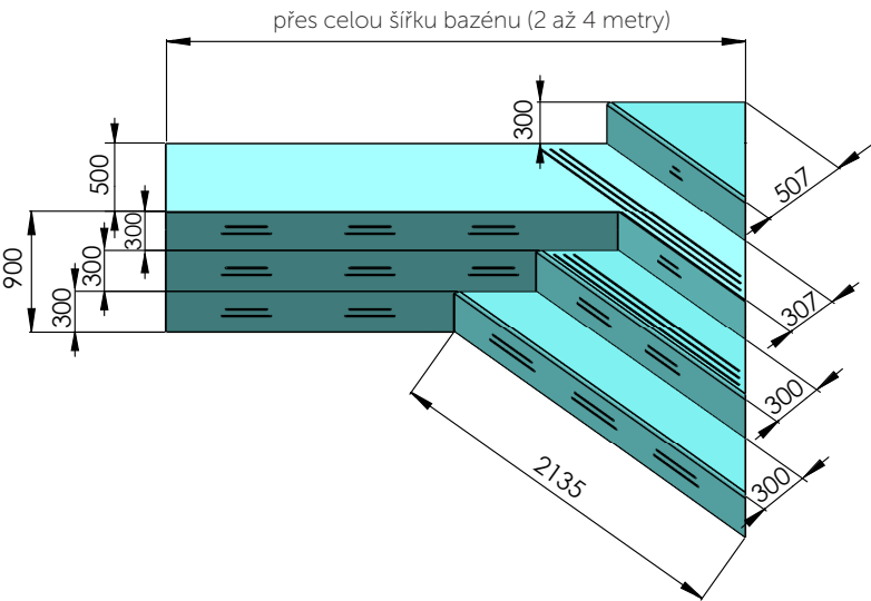
Schody rovné přes roh s lavicí 4-stupňové pro hloubku 1,5 m přes celou šířku bazénu (2 až 4 metry)
