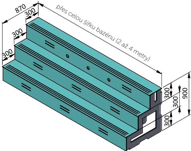
Schody obdélníkové 3-stupňové pro hloubku 1,2 m přes celou šířku bazénu (2 až 4 metry)
