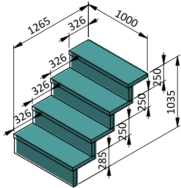
Schody X-AIR 4-stupňové pro hloubku 1,2 m pravé provedení: 2B04-01-SD084 levé provedení: 2B04-01-SD074
